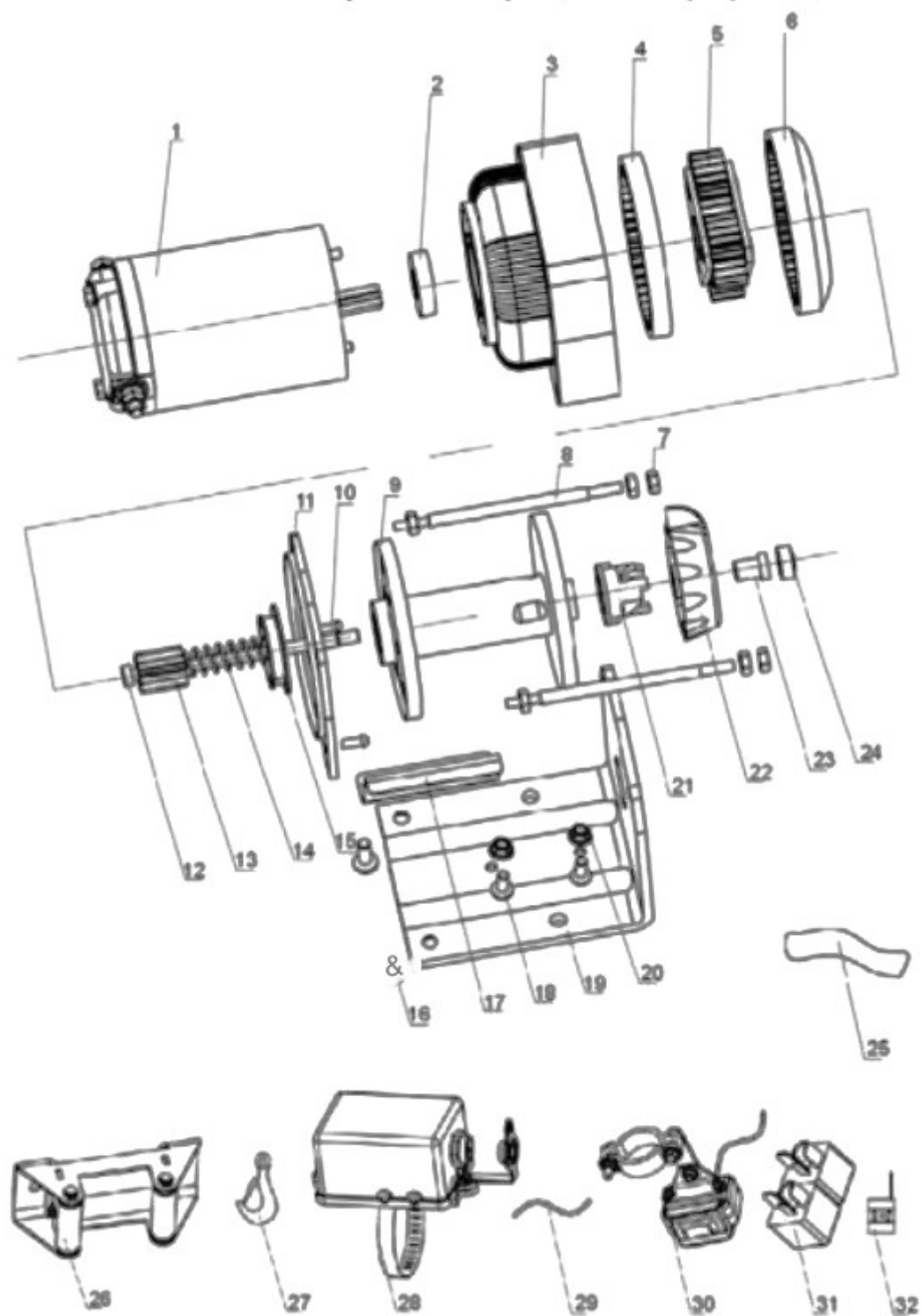
Elektrický ATV naviják rozložený výkres
