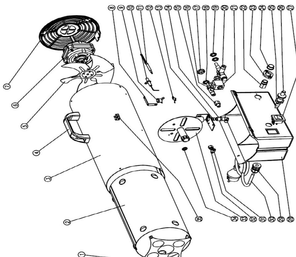
MONTÁŽNÍ VÝKRES
